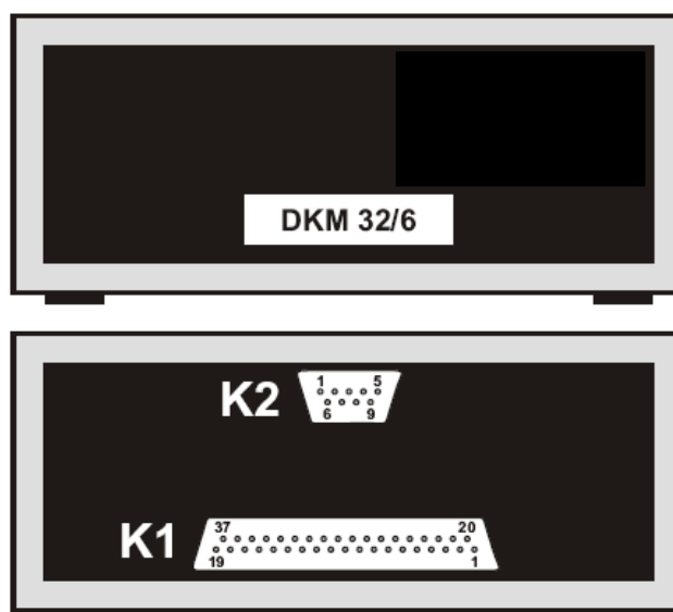
Slika br. 1: Diodno kodna matrica DKM 32/6
